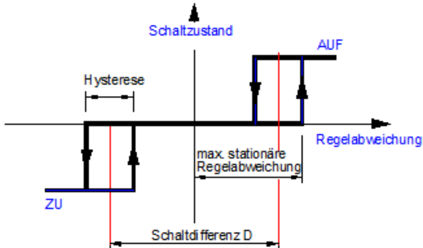
Bild 4: Schaltpunkte des 3-Punktreglers
