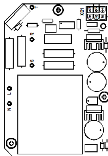
Bild 2: Power supply
